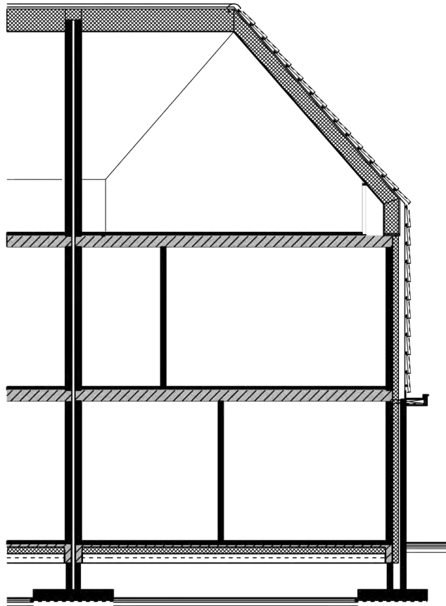
doorsnede 1:100
