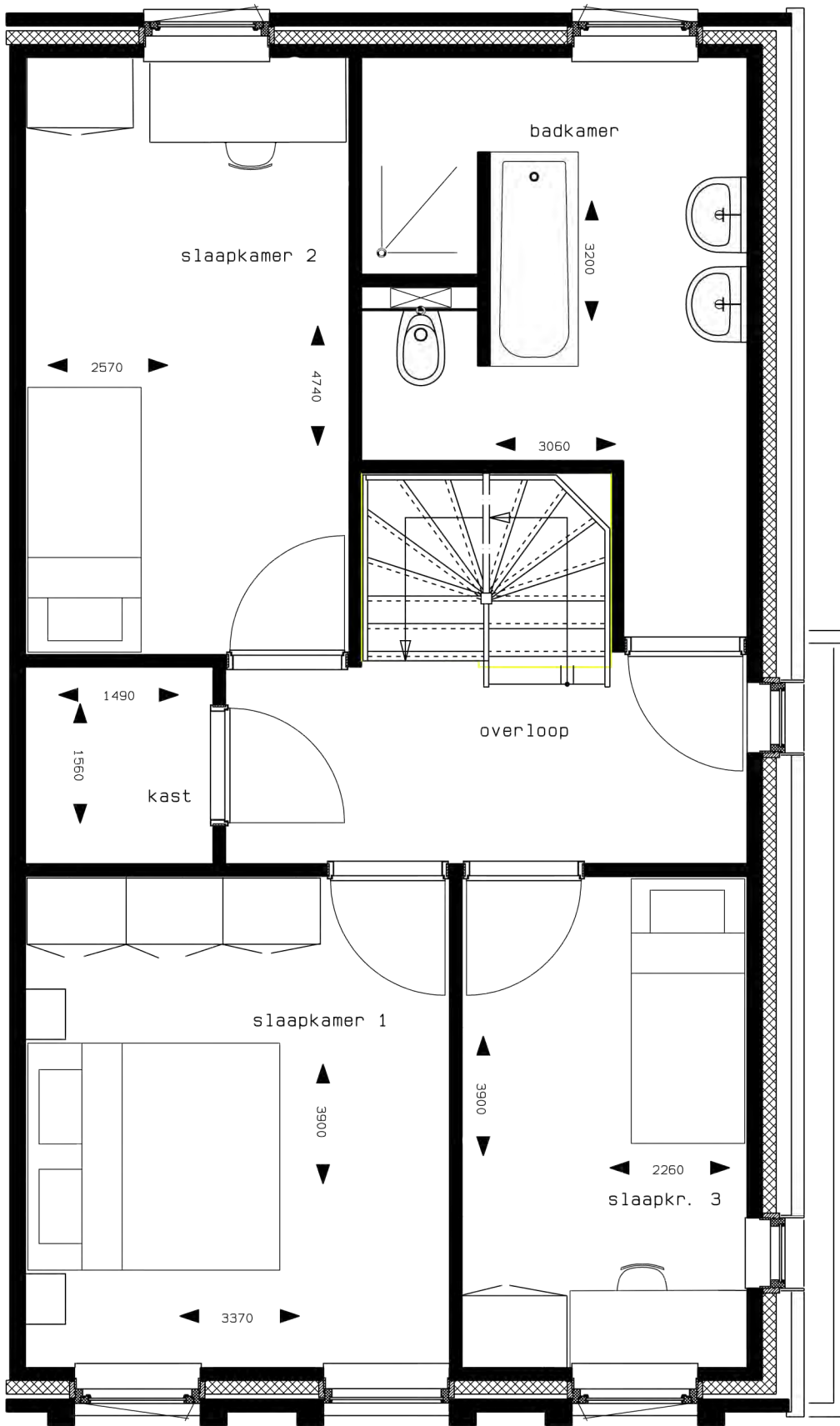
plattegrond verdieping 1:50
