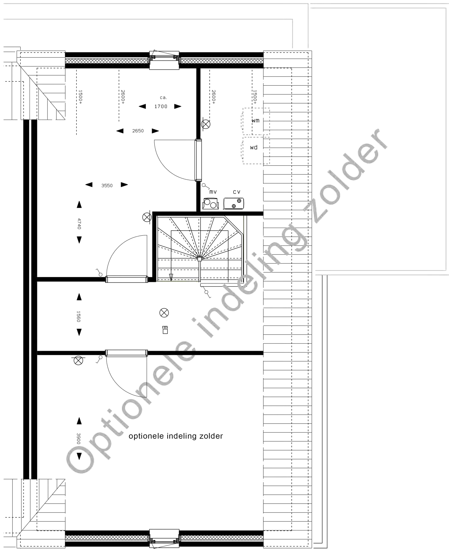
plattegrond zolder 1:50
